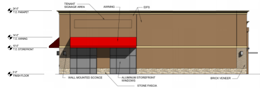
2 WEST ELEVATION SCALE: 1:20
