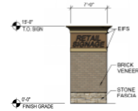
5 SIGN ELEV. SCALE: 1:20
