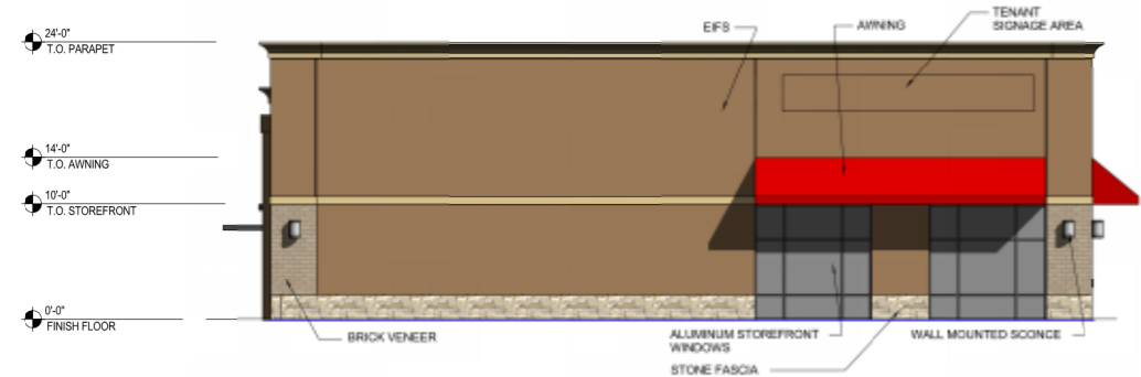
4 EAST ELEVATION SCALE: 1:20
